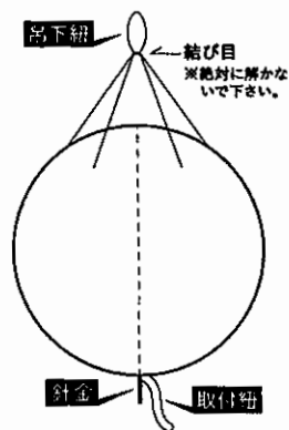
取付紐部分 拡大図
